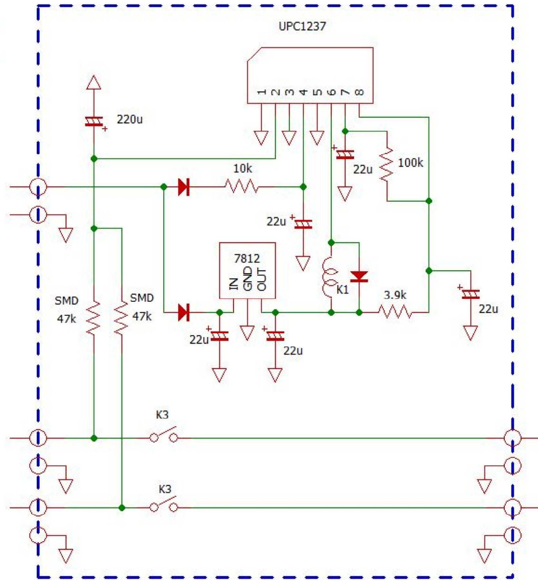
SoftStart回路に使用したSpeaker Protect Module(完成品)のオリジナル回路
